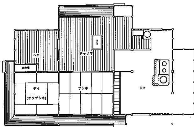
今回の復元 角屋 19世紀中頃
